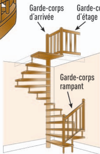
Escalier d'angle à trémie carré
